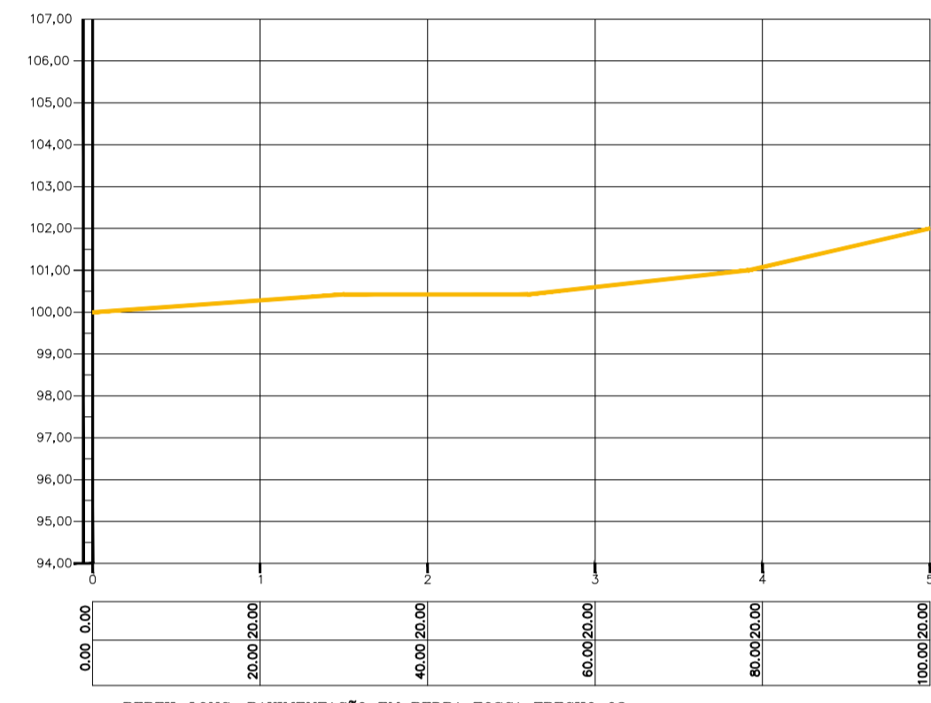
PERFIL LONG. PAVIMENTAÇÃO EM PEDRA TOSCA TRECHO 02 ESCALA: 1/750 V=1/80
